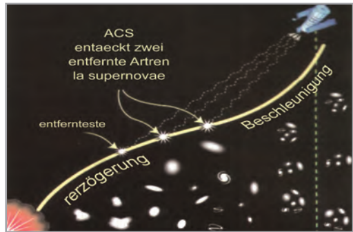
Diese Abbildung zeigt, dass sich das Universum erweitert
