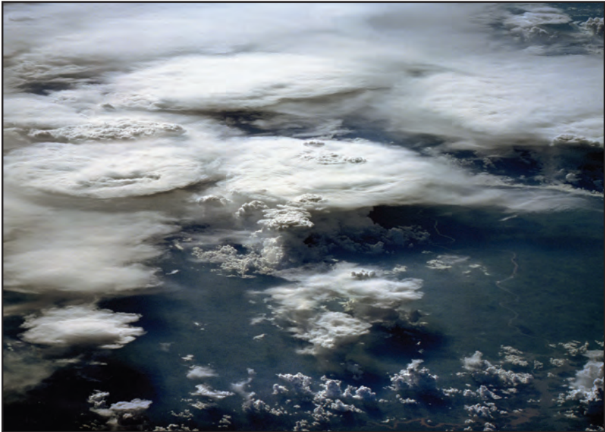
Eine Gewitterwolke. Dieses Bild wurde vom NASA Satelliten aufgenommen. Es ist so, als ob eine unsichtbare Hand die Haufenwolken zur Konvergenzzone treibt.
