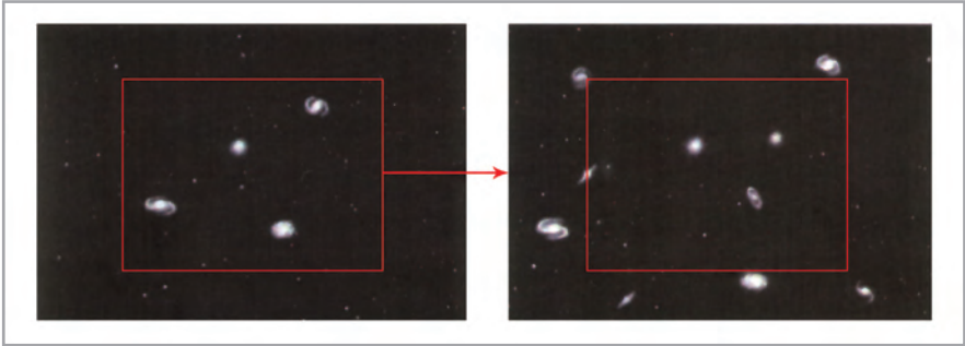
Diese Abbildung zeigt, dass die Abstände zwischen Galaxien oder Blöcken der Galaxien fortwährend zunehmen und sich das Universum folglich erweitert
