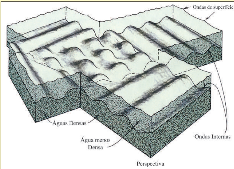
Figura 16: Ondas internas na interface entre duas camadas de água de densidades diferentes. Uma é densa (a mais baixa), a outra é menos densa (a superior). ( Oceanography [Oceanografia], Gross, p. 204.)
