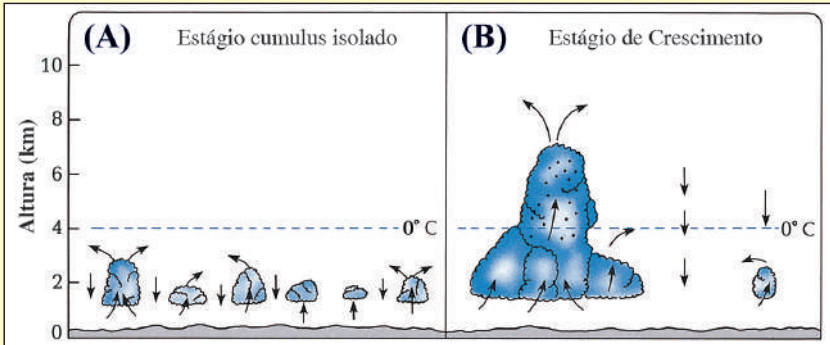
Figura 19: (A) Pequenos pedaços isolados de nuvens (nuvens cumulus). (B) Quando as pequenas nuvens se unem, as correntes de ar ascendentes dentro da nuvem maior aumentam, de modo que a nuvem é empilhada. Gotas de água são indicadas por · ( The Atmosphere [A Atmosfera], Anthes e outros, p. 269.)
